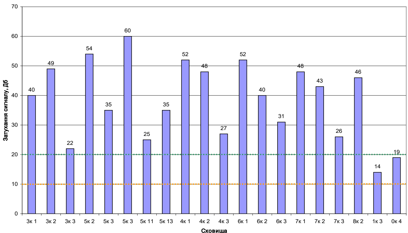
Рис. 1. Діаграма затухання радіосигналів у приміщеннях будівлі восьмйярусного фондосховища НБУВ
