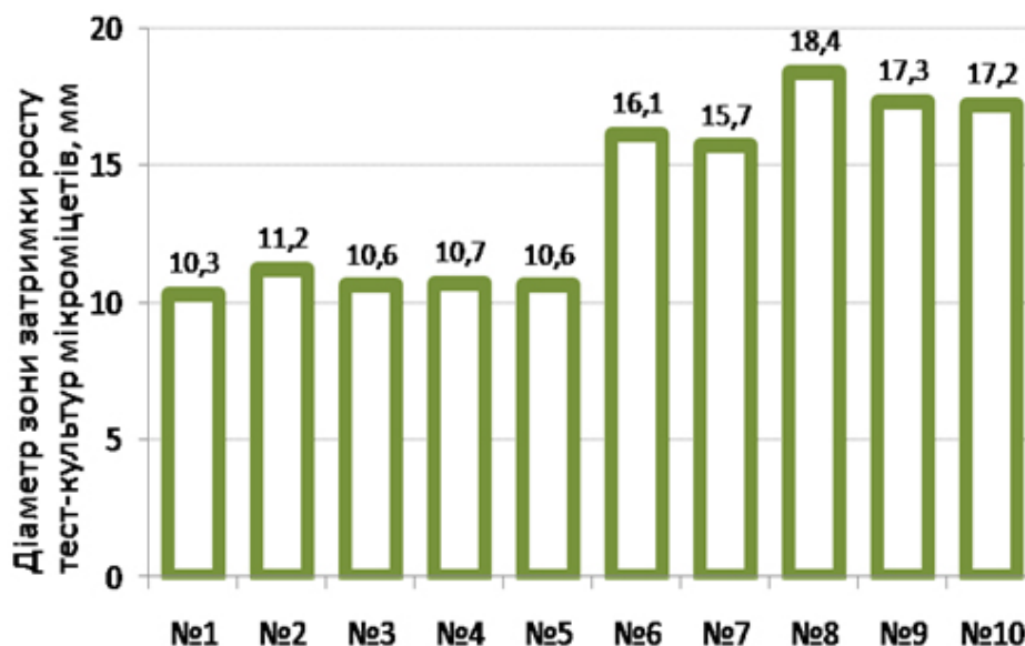
Рис. 1. Середнє значення зон затримки росту тест-культур мікроміцетів за впливу композитних гуанідиновмісних олігомерів з додаванням срібла та міді
