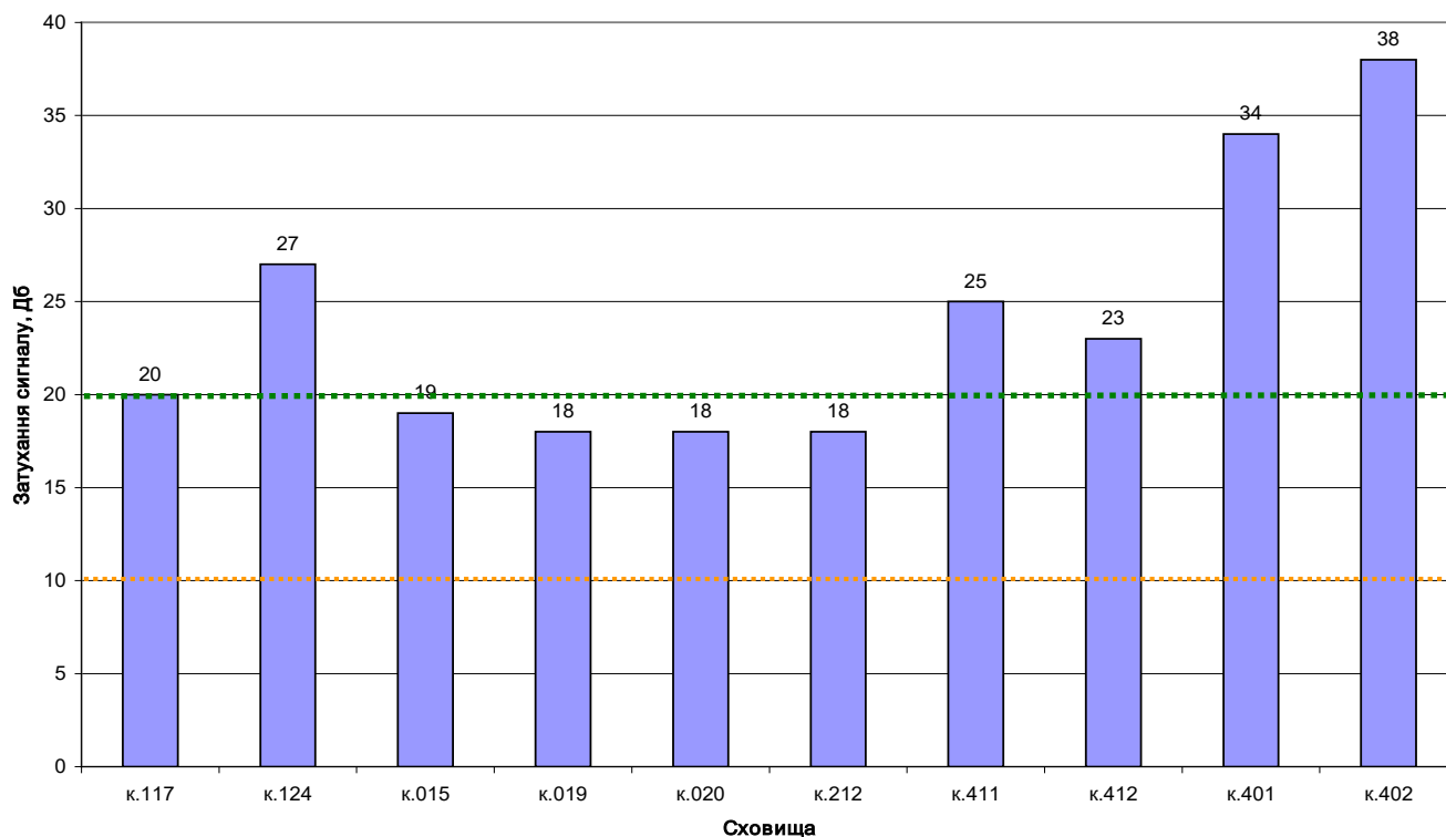
Рис. 2. Діаграма затухання радіосигналів у фондосховищах чотириповерхового корпусу НБУВ
